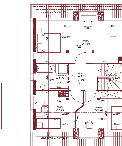
Piętro
